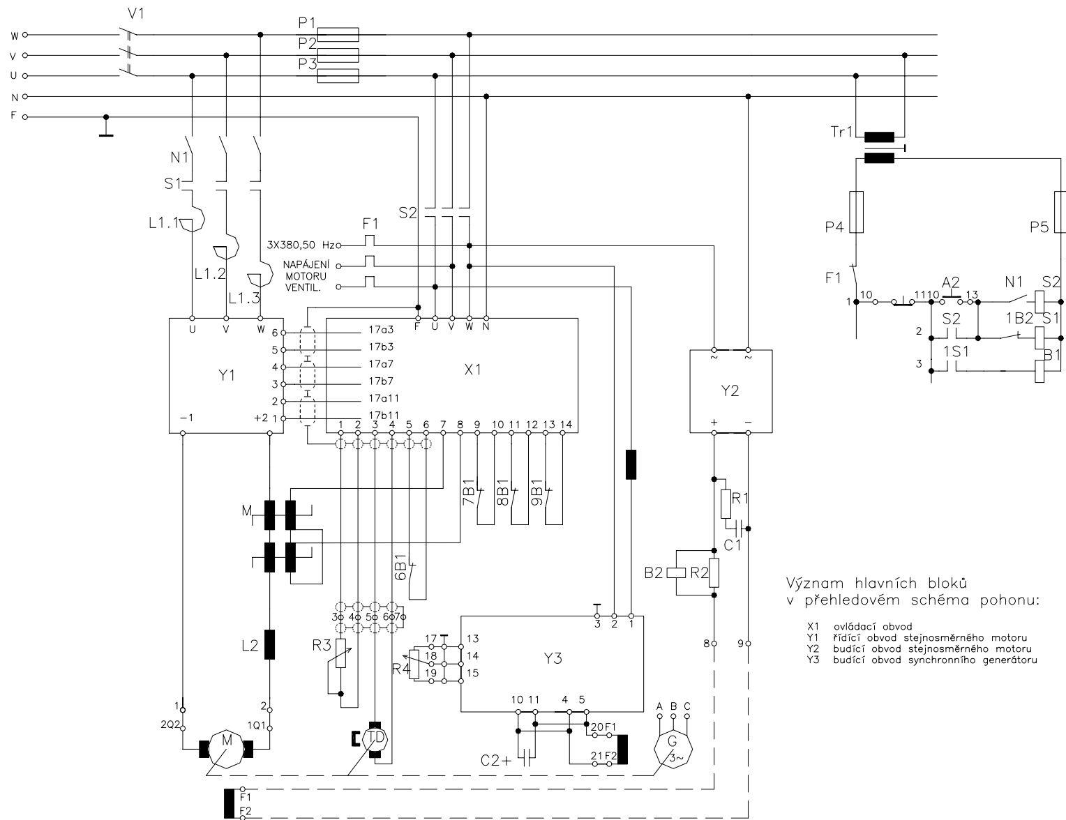
Obr. P1.1 Přehledové schéma pohonu motor–generátoru
