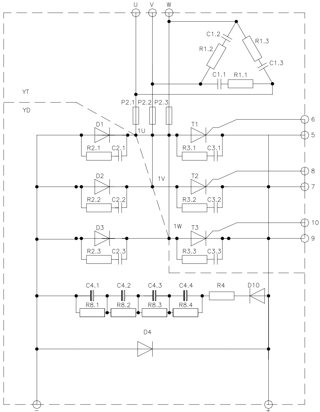
Obr. P2.1 Schéma zapojení výkonového bloku polořízeného 6pulzního usměrňovače
